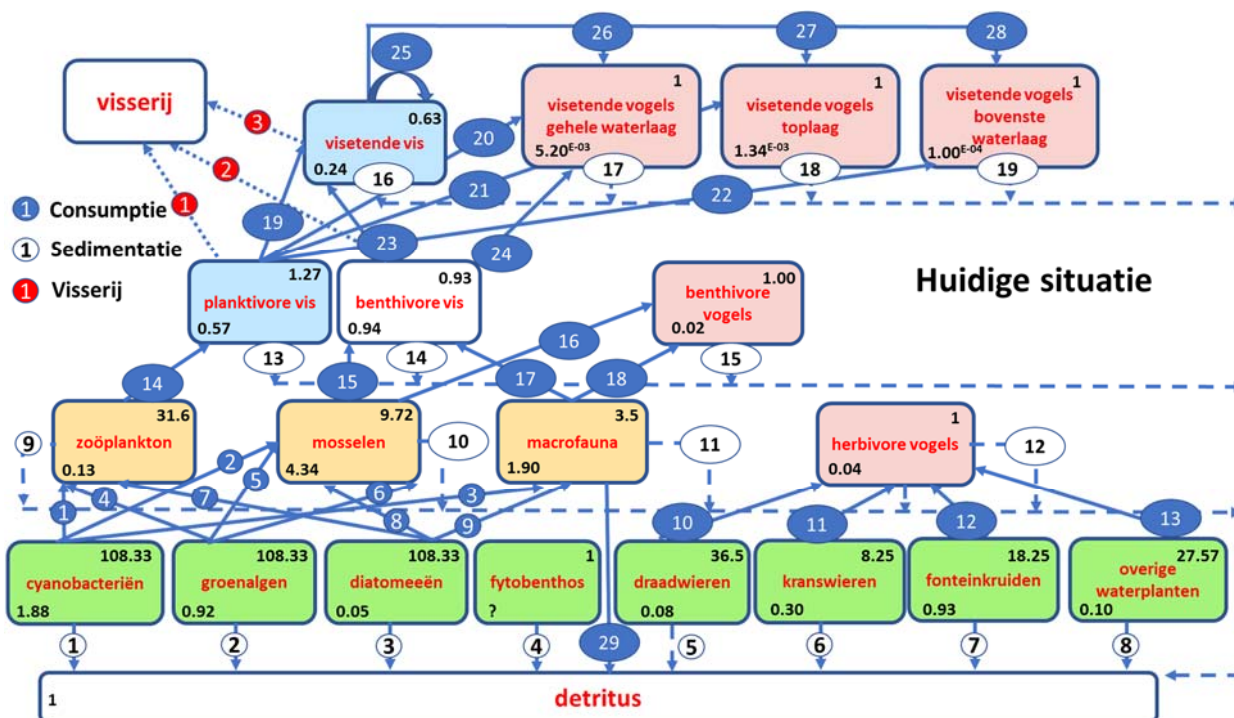
Figuur 6-1 Statisch voedselwebmodel van het Markermeer in de huidige toestand zoals gemodelleerd met behulp van Ecopath. In elke component van het voedselweb is links onder de biomassa (g/m 2 ) en rechtsboven de productie (g/m 2 /jaar) gegeven. De cijfers op de pijlen verwijzen naar consumptie (zie tabel 6.1) en sedimentatiesnelheden (tabel 6.2) en visserijvangst (tabel 6.3).
